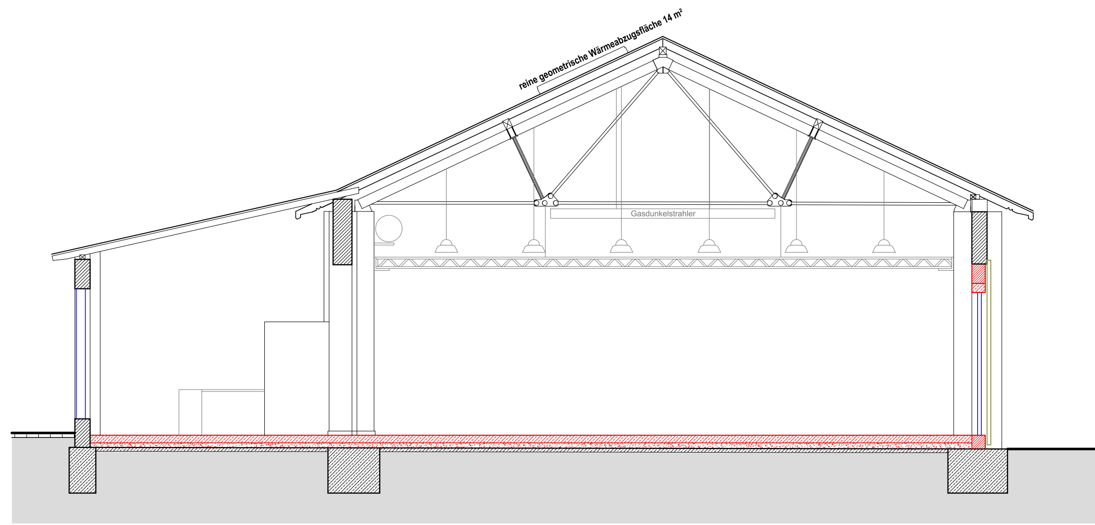
Schnitt A-A
